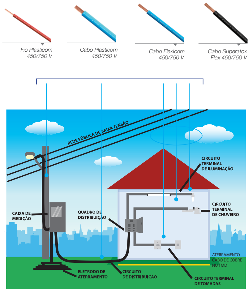
FIGURA 1 · APLICAÇÕES EM INSTALAÇÕES RESIDENCIAIS
