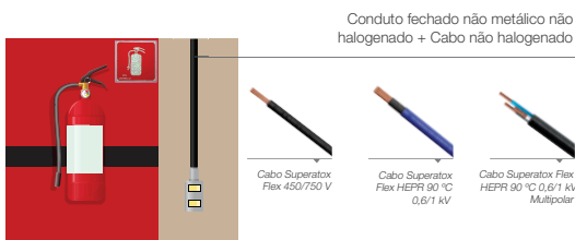
FIGURA 13 · LINHAS APARENTES COM CONDUTOS FECHADOS NÃO METÁLICOS EM LOCAIS DE AFLUÊNCIA DE PÚBLICO
