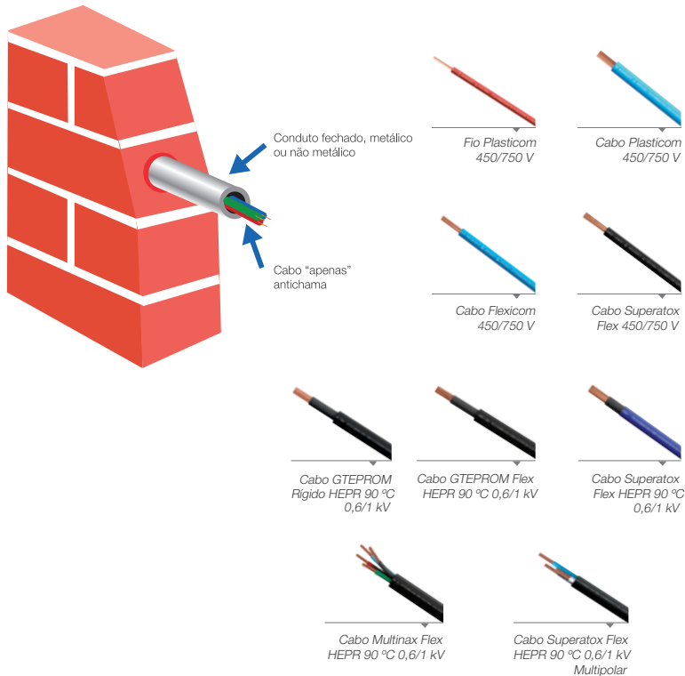
FIGURA 10 · LINHAS EMBUTIDAS EM LOCAIS DE AFLUÊNCIA DE PÚBLICO
