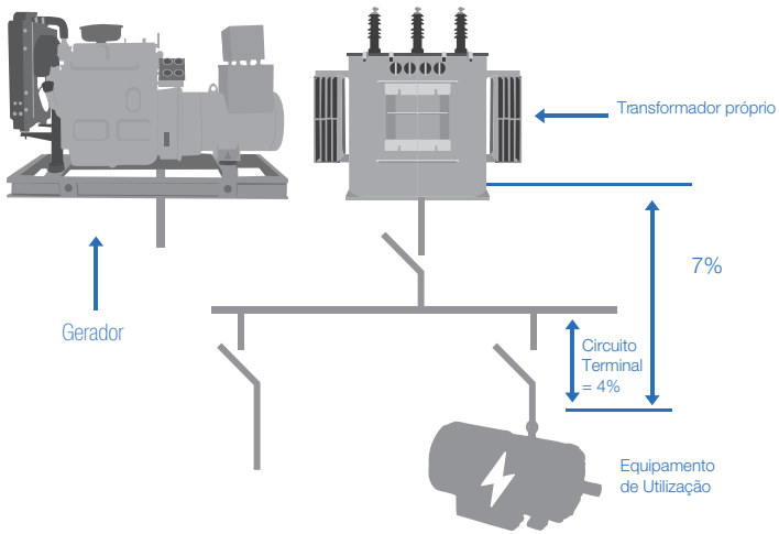
FIGURA 9 · QUEDA DE TENSÃO MÁXIMA EM INSTALAÇÃO (FORNECIMENTO EM TENSÃO SECUNDÁRIA)
