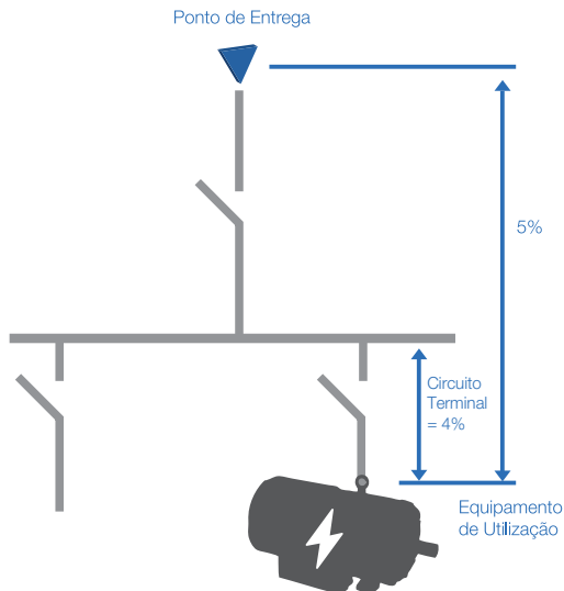
FIGURA 9 · QUEDA DE TENSÃO MÁXIMA EM INSTALAÇÃO (FORNECIMENTO EM TENSÃO SECUNDÁRIA)
