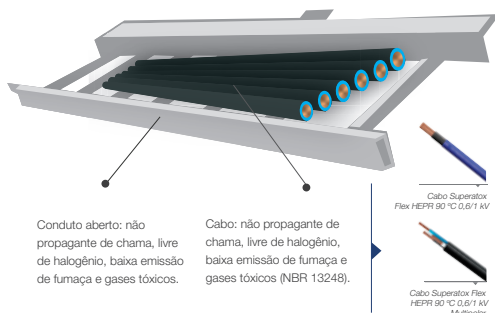
FIGURA 12 · LINHAS APARENTES COM CONDUTOS FECHADOS METÁLICOS EM LOCAIS DE AFLUÊNCIA DE PÚBLICO
