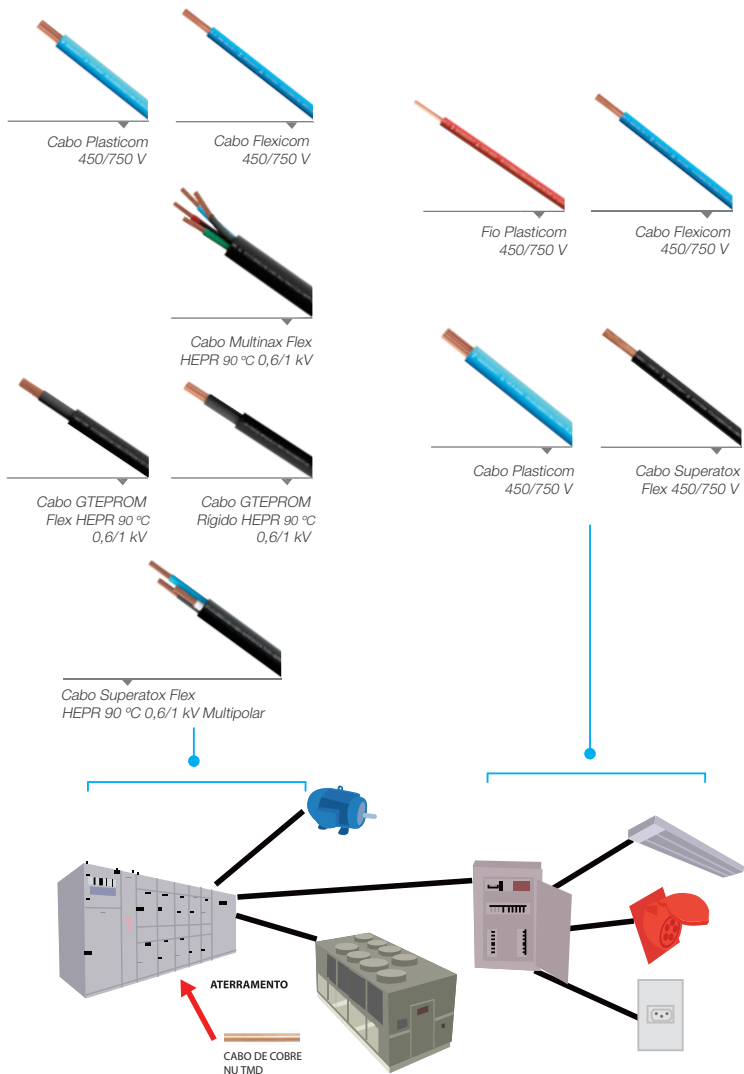
FIGURA 3 - APLICAÇÕES EM INSTALAÇÕES COMERCIAIS DE GRANDE PORTE E INDUSTRIAIS
